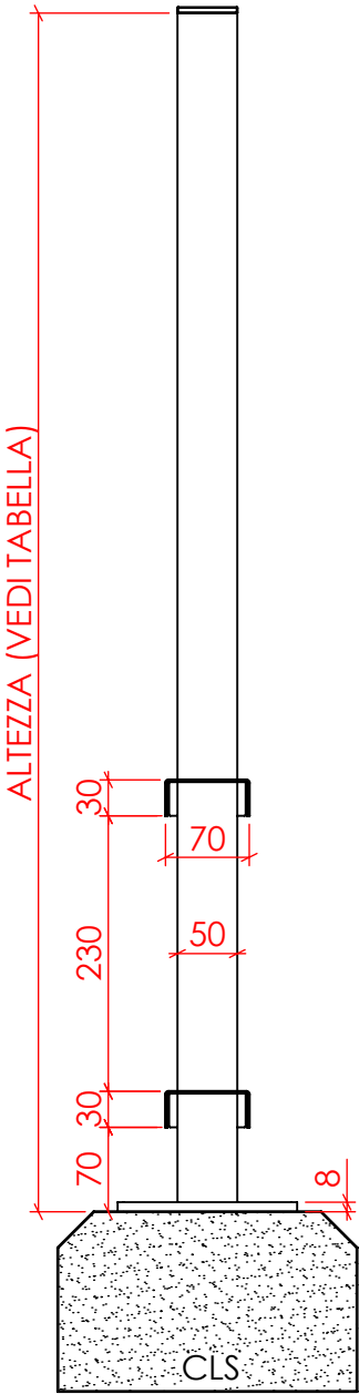
SEZIONE B-B
