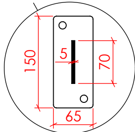
DETAGLIO MONTANTE
