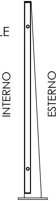
SEZIONE B-B 2° POSIZIONE MONTAGGIO
