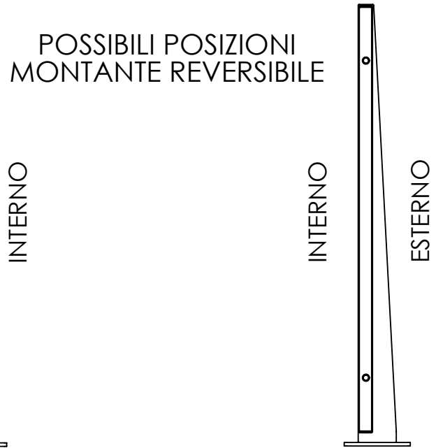
SEZIONE B-B 2° POSIZIONE MONTAGGIO
