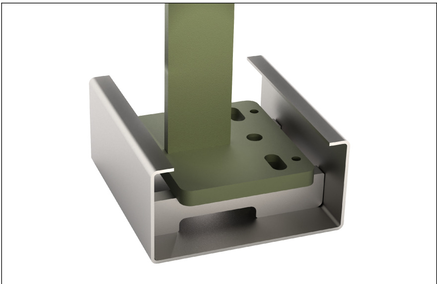
Dettaglio piastra per fissaggio dentro canale Noè
