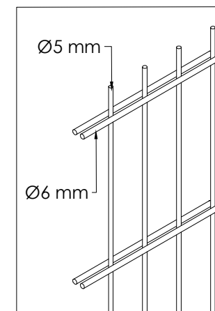
DETTAGLIO TAMPONATURA
